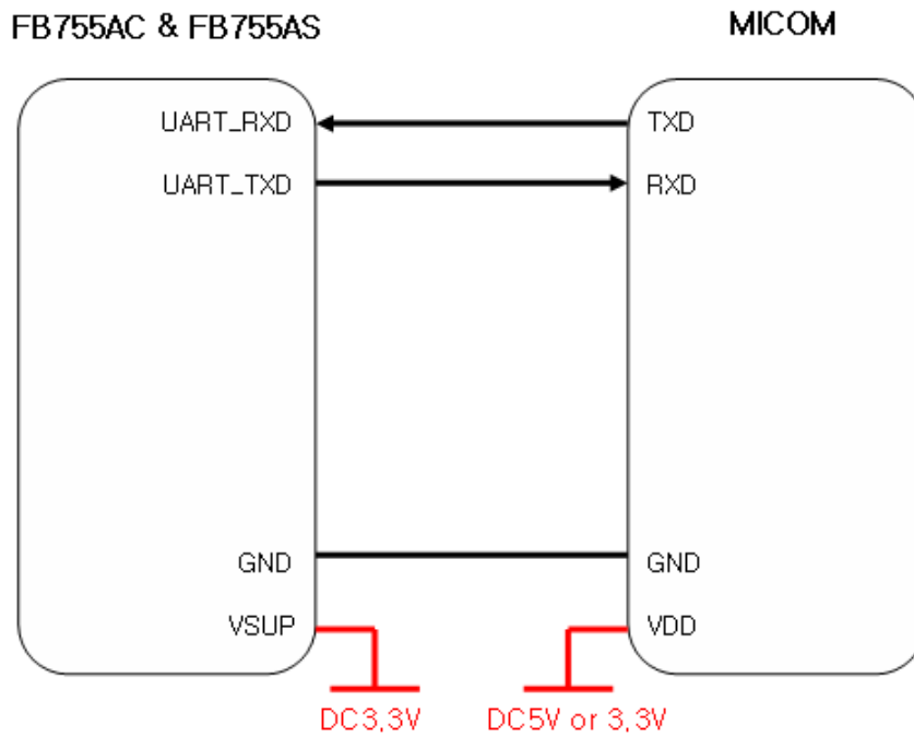
<그림 5-1 흐름제어 사용하지 않을 때의 핀 연결도>
