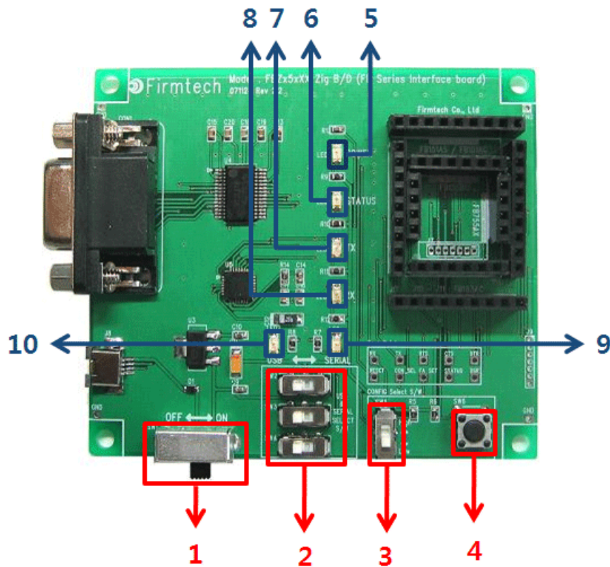
<그림 6-1 FB755AX Interface Board(Jig Board)>
